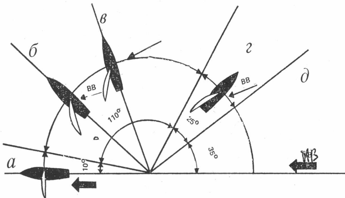
Рис.9. Курсы и галсы относительно ветра:
