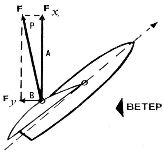
Рис.4. Подъемная сила и сопротивление паруса (аэродинамические силы)
