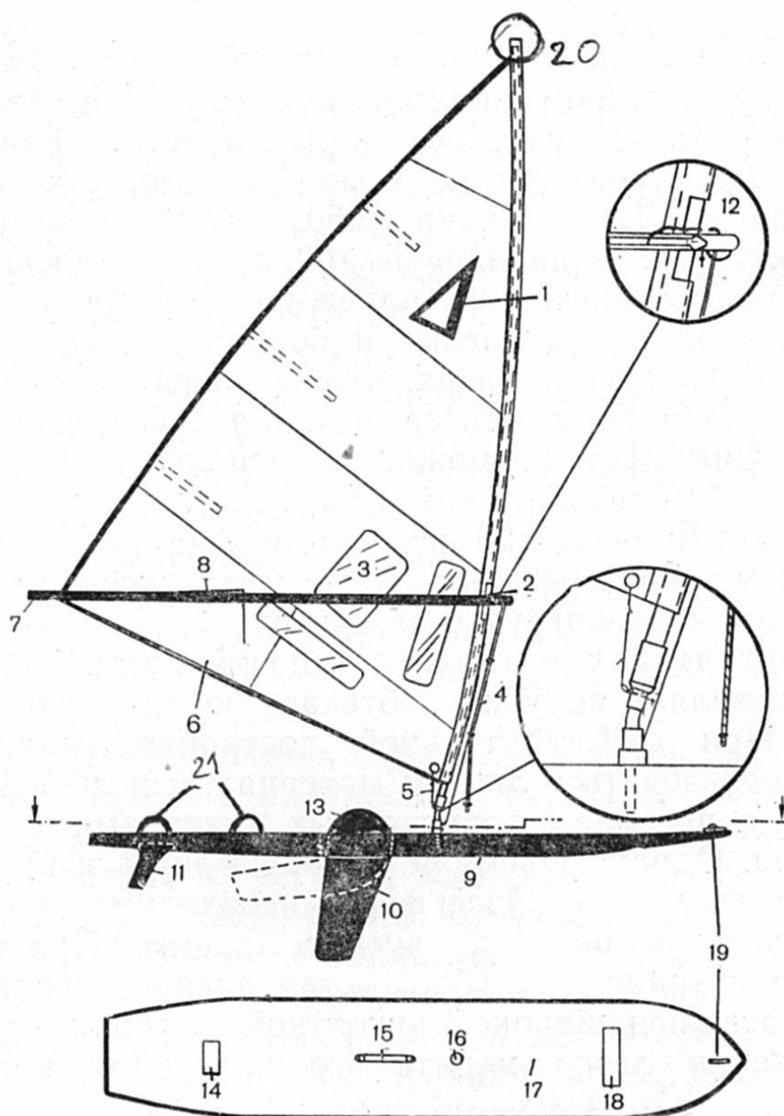
Рис 1. Доска для занятия виндсерфингом в сборе.
