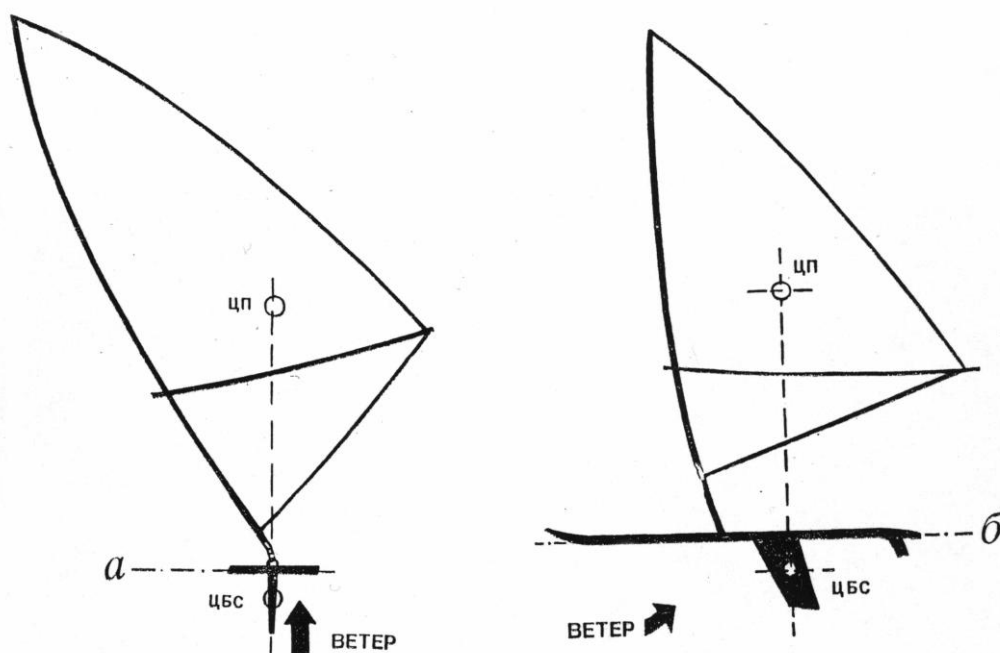
Рис.10. Принцип управления доской.
