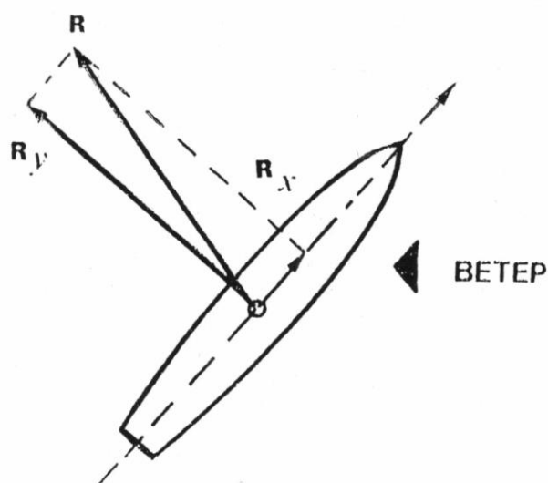
Рис.6. На курсе бейдевинд боковая гидродинамическая сила ( R_y ) значительно больше силы тяги ( R – равнодействующая гидродинамических сил; R_x – гидродинамическое сопротивление).
