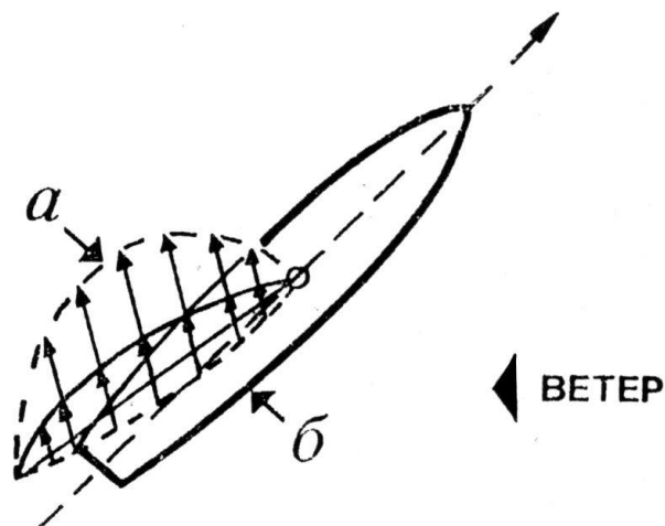
Рис.5. Разрежение с подветренной стороны паруса (а) и избыточное давление на наветренной его стороне(б).
