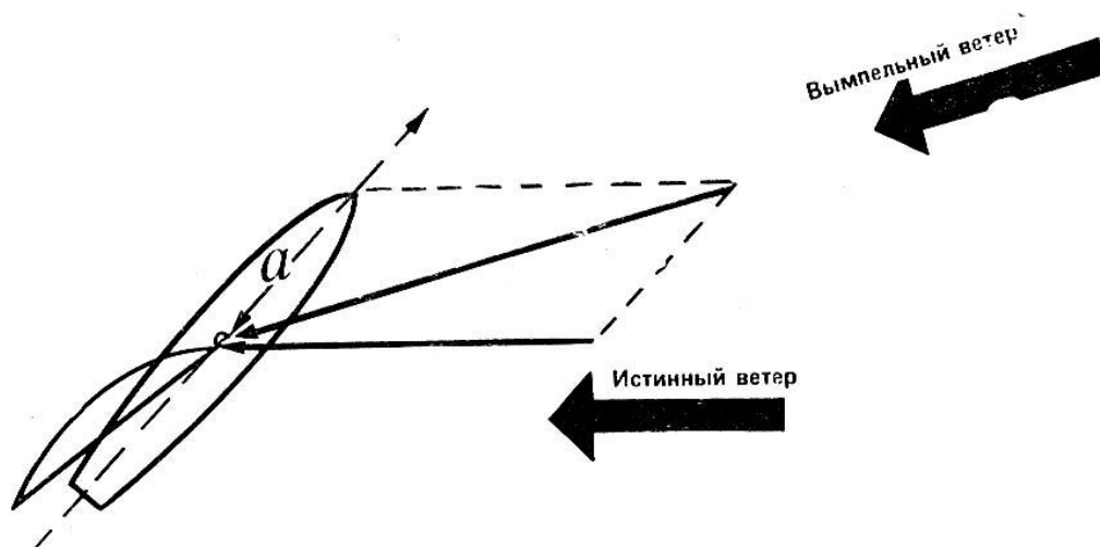
Рис.8. В движении истинный ветер в значительной мере «искажается» и предстает как курсовой ветер: а – курсовой ветер.
